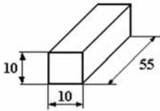
Şekil 2. T/M Numunelerin şekli ve boyutu
