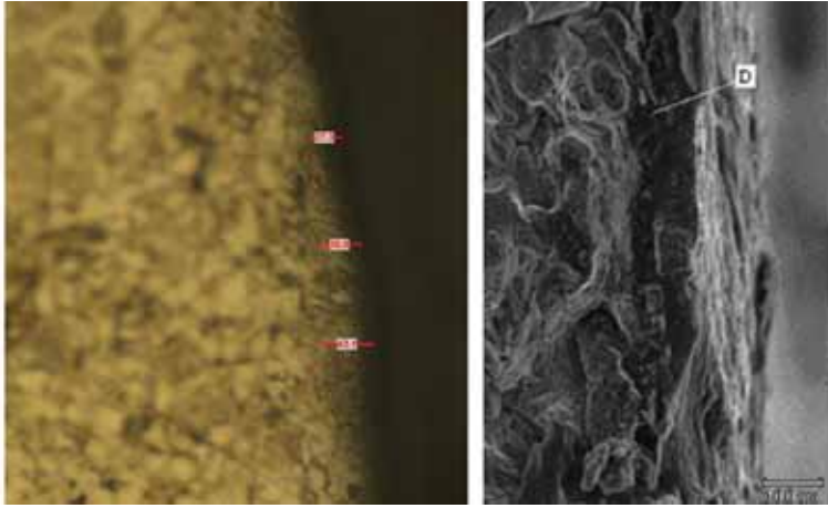
Şekil 9. P+20A+Isıl İşlem uygulanmış TM çelik numunenin görünümü
