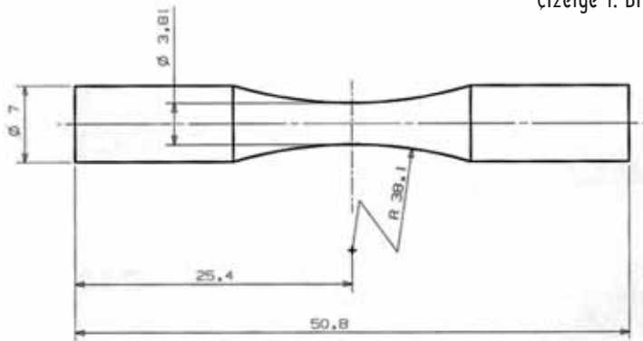
Şekil 3. Deneylerde kullanılan yorulma numunelerinin şekil ve boyutları
