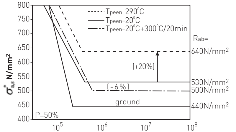
Şekil 1. Farklı sıcaklıkta bilyeli dövülmüş ve dövme işlemi yapılmamış AISI 4140 çeliğinden imal edilmiş numuneler için S-N eğrileri [6]
