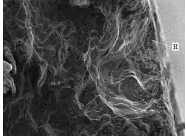
Şekil 7. P+32A+Isıl İşlem uygulanmış TM çelik numunenin yorulma kırık görünüsü (x750)
