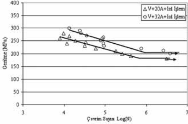
Şekil 5. V+20A+Isıl İşlem ve V+32A+Isıl işlemlerine tabi tutulmuş TM çelik numunelerin S-N eğrileri
