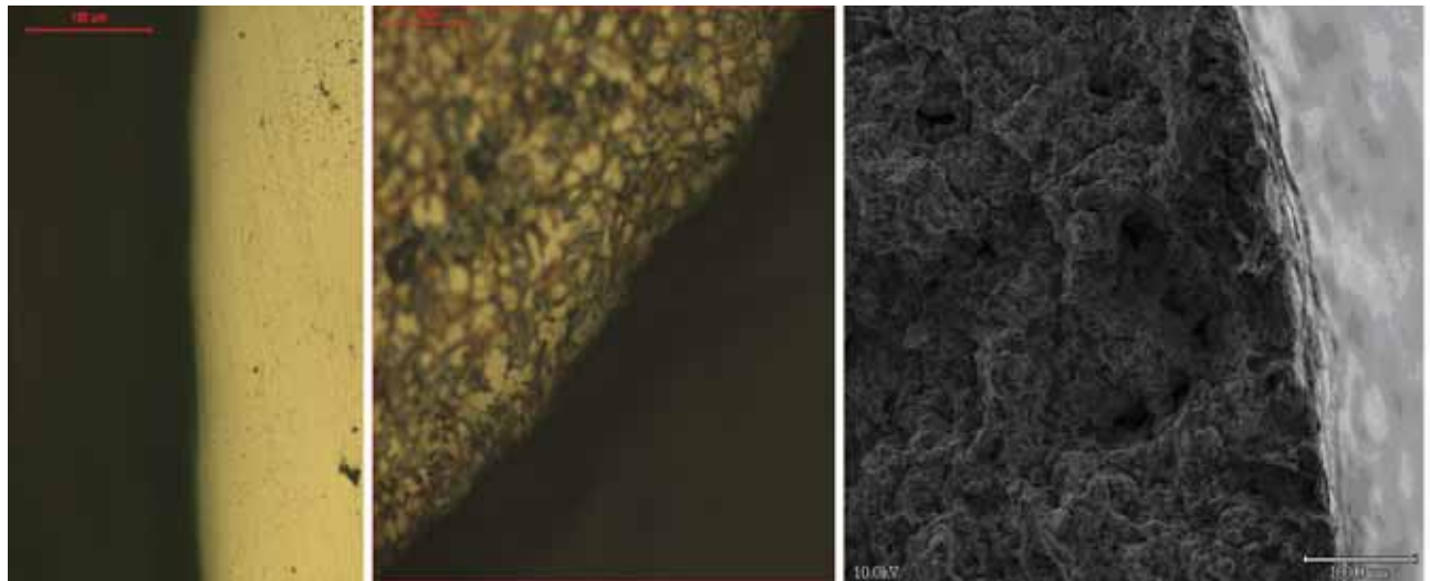
Şekil 10. V+20A+Isıl İşlem uygulanmış TM çelik numunenin değişik görünüşleri
